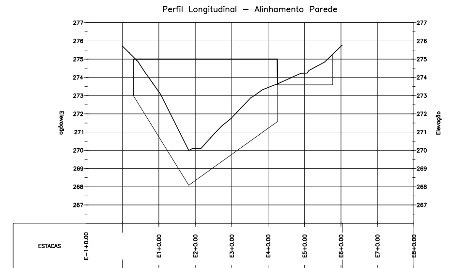
01 PERFIL LONGITUDINAL DA PAREDE ESCALA = 1:1000
