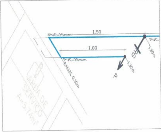
DISTRIB. ÁREA DE SERVIÇO ISOMÉTRICO esc: 1:25
