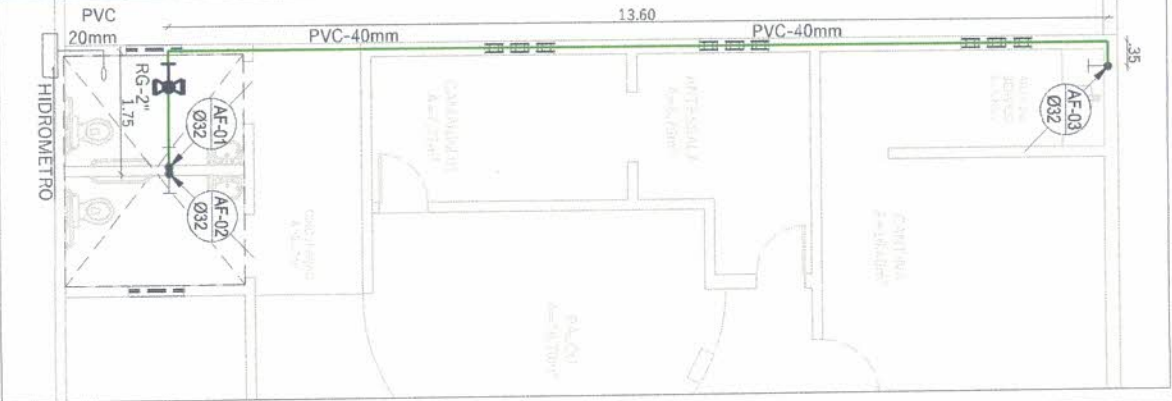
DISTRIB. ÁREA DE SERVIÇO PLANTA BAIXA esc: 1:40
