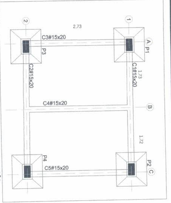
PLANTA DE FUNDAÇÃO esc: 1:40
