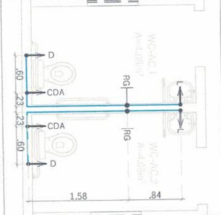
DISTRIB. BANHEIROS PLANTA BAIXA esc: 1:40
